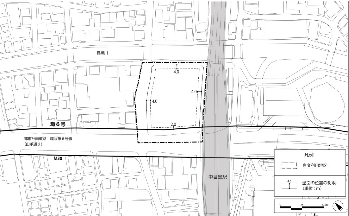
壁面の位置の制限図
