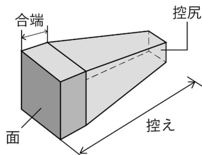
図 3-20 間知ブロックの各部名称
