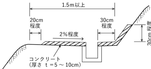
図 3-65 小段排水工
