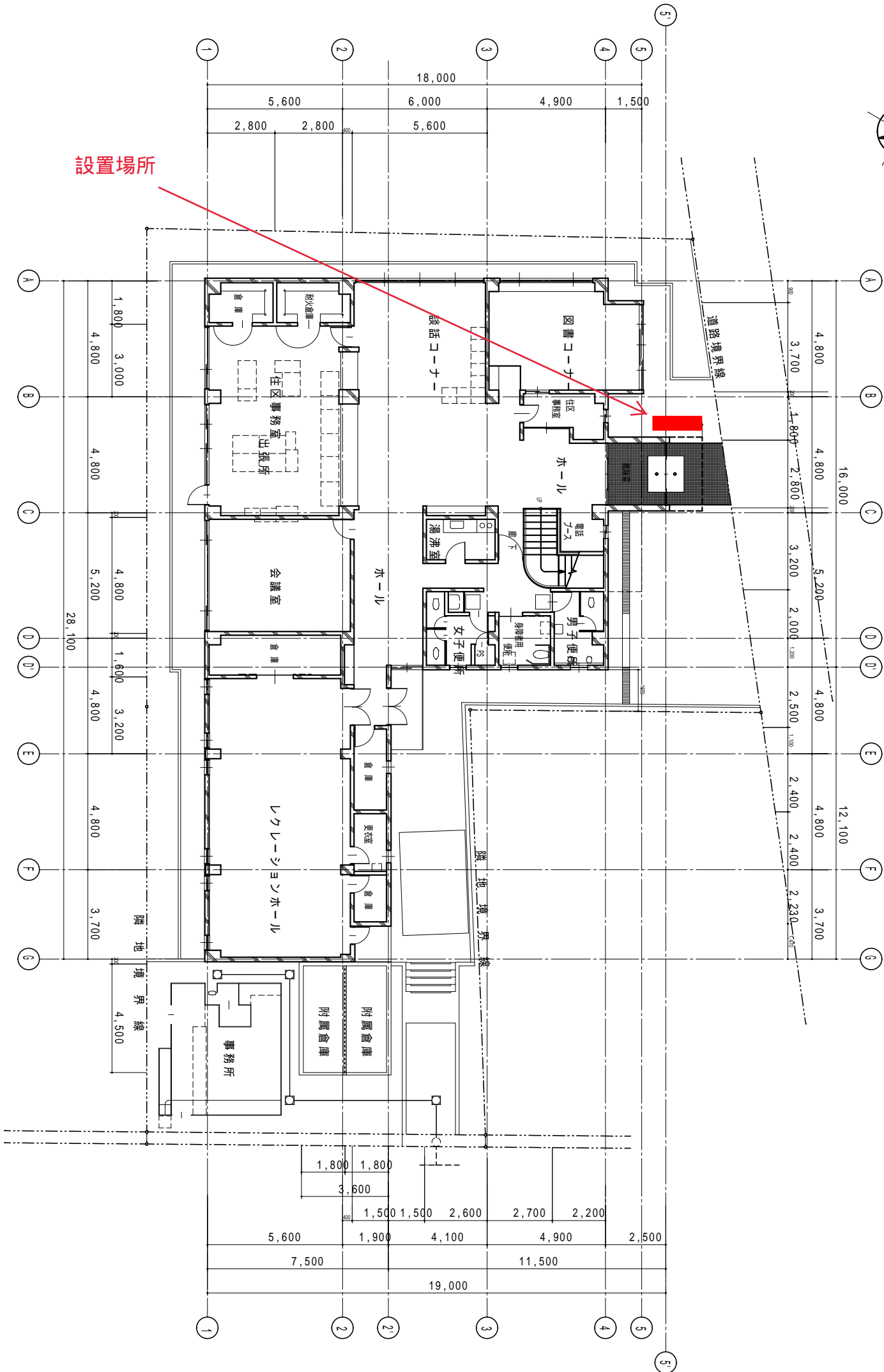
大岡山西住区センター 1階平面図 S=1:100
