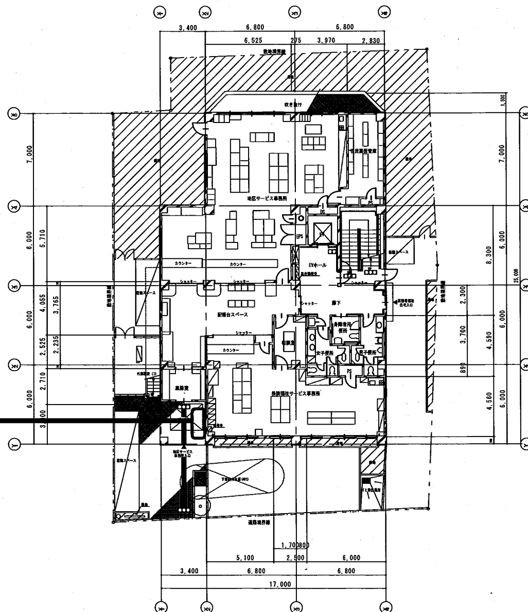
西部地区サービス事務所 配置図・1階平面図 S=1:100
