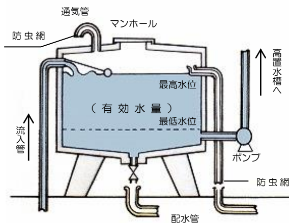
受水層の構造
