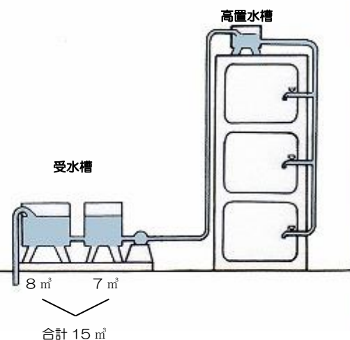
簡易専用水道の該当例
