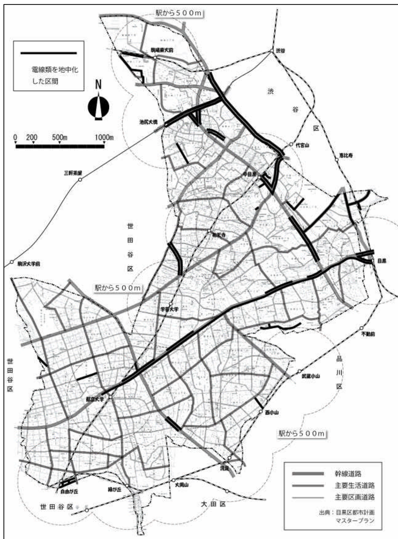
図 2-3 電線類を地中化した区間
