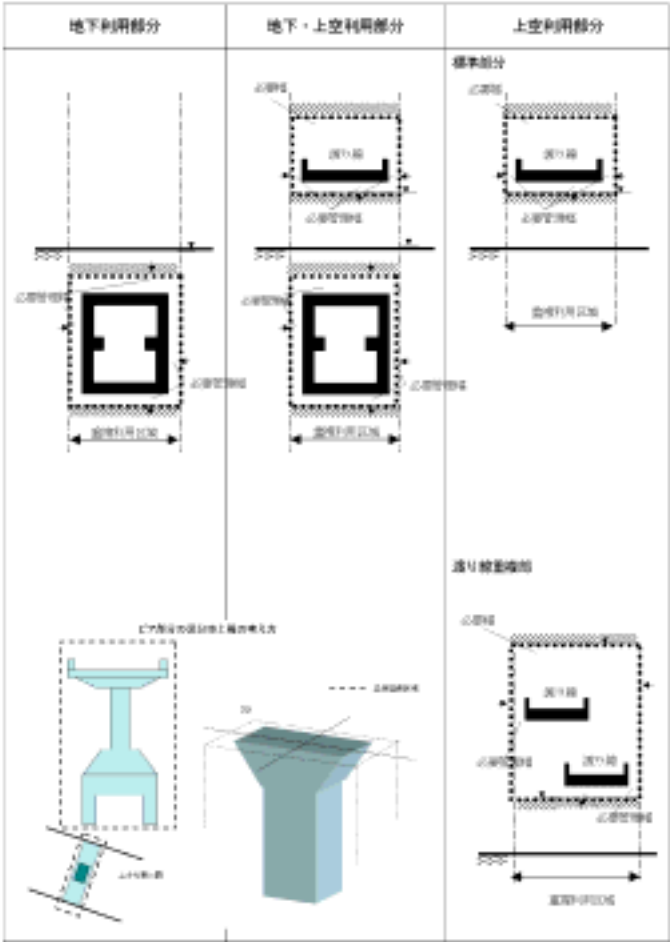
立体道路区域決定イメージ図
